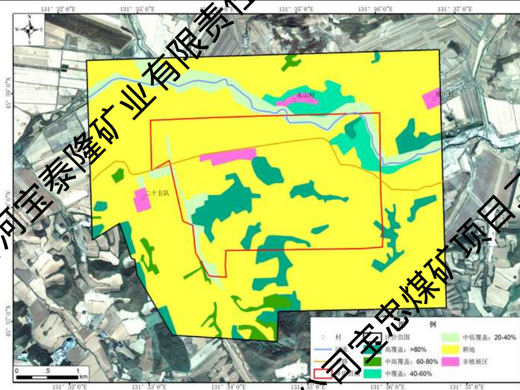
图 4.3-4 评价区及井田植被覆盖度解译图
